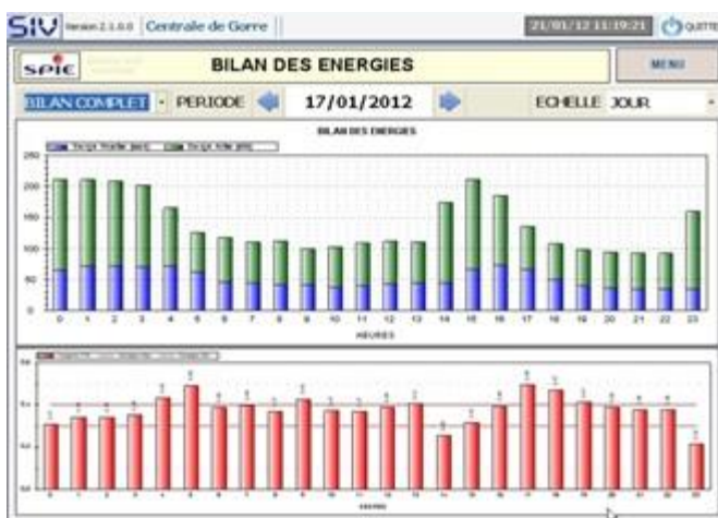
Bilan d'énergie au PDL permettant de vérifier le respect du bandeau de tangente
